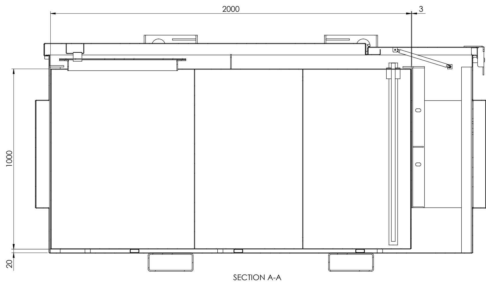
SECTION A-A
