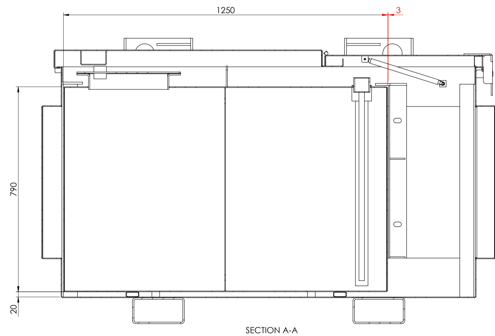
SECTION A-A
